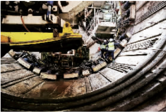
检查尾盾压千斤顶。
