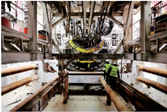
盾构机内部。
