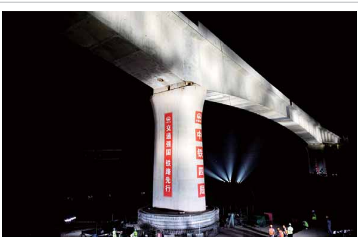
这是合安高铁肥西联络线跨合武铁路100米连续梁转体施工现场(9月9日摄)。9月9日,由中铁四局承建的合安高铁肥西联络线跨合武铁路100米连续梁成功转体,标志着合安高铁控制性重难点工程全部完成。合安高铁自新合肥西站引出,终至新安庆西站,设计时速350公里,预计2020年建成通车。
